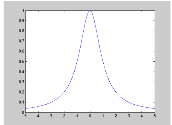
Figura 2.1 Curva de Agnesi
