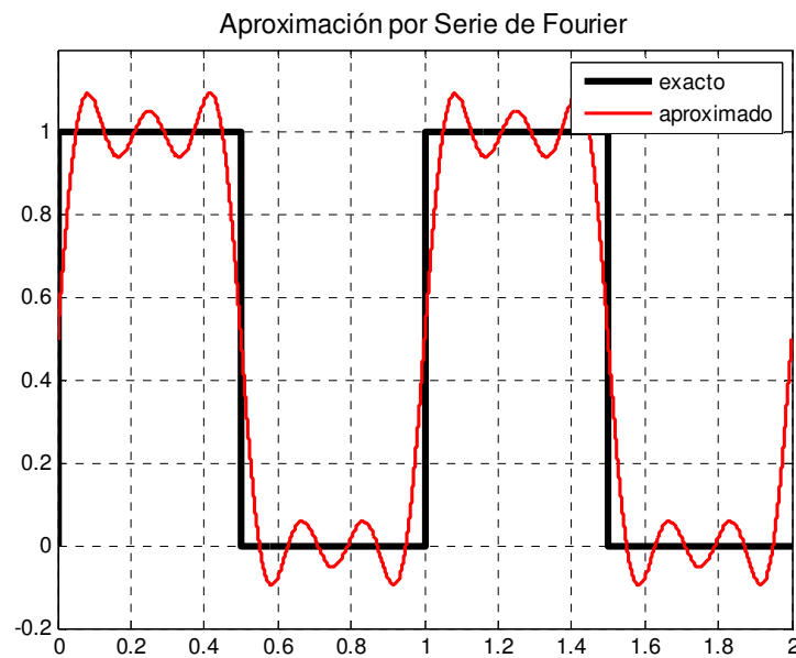
Figura 3.1. Aproximación del tren de pulsos obtenida al ejecutar fourier_aprox(2) con N=5 .
