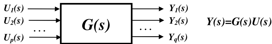
Figura 4.2.- Diagrama de Bloques de un sistema con p entradas y q salidas
