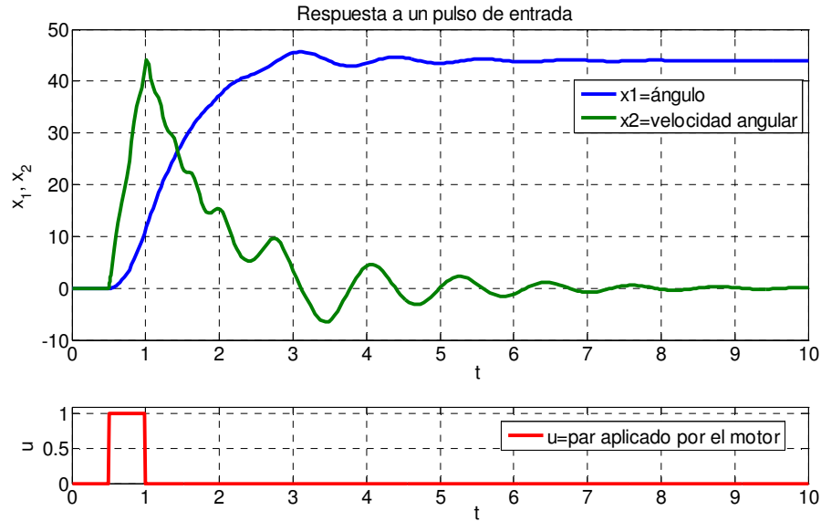
Figura 5.6.- Respuesta de la varilla a un pulso de par aplicado por el motor.
