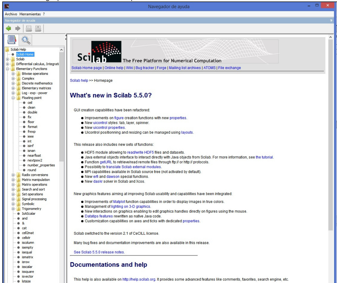
Figura 1.2.- Ventana inicial del Navegador de ayuda de Scilab
