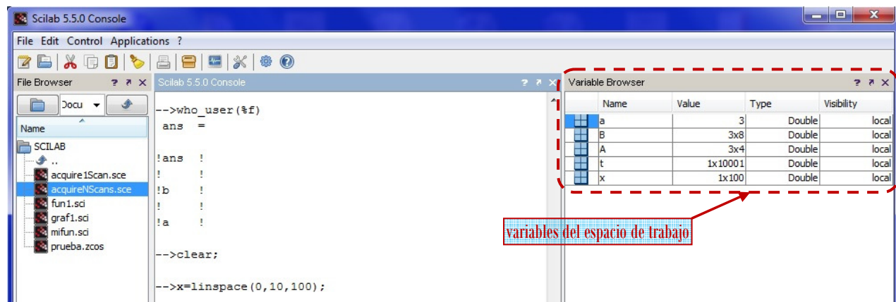
Figura 1.3.- navegador de variables mostrando el espacio de trabajo de Scilab.
