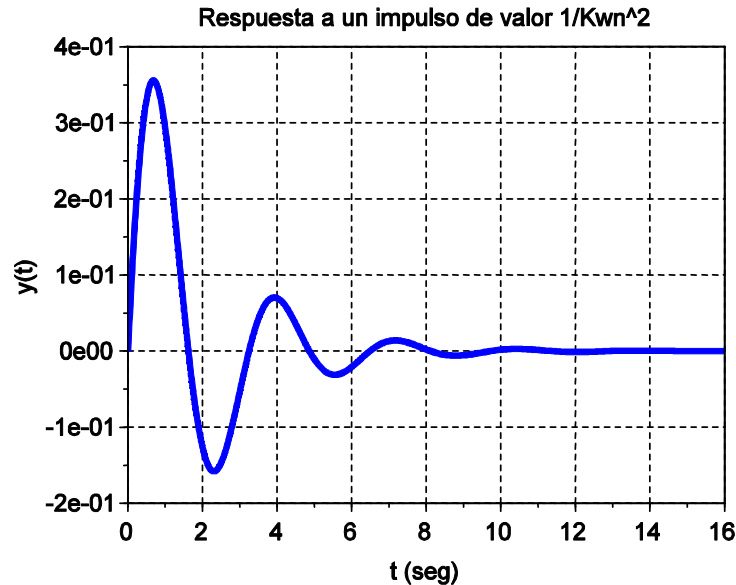
Figura 10.6.- Respuesta del sistema de 2º orden a un impulso \delta(t) / K\omega_n^2 .
