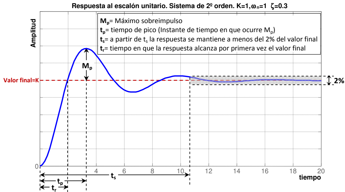
Figura 10.2.- Especificaciones de respuesta transitoria.
