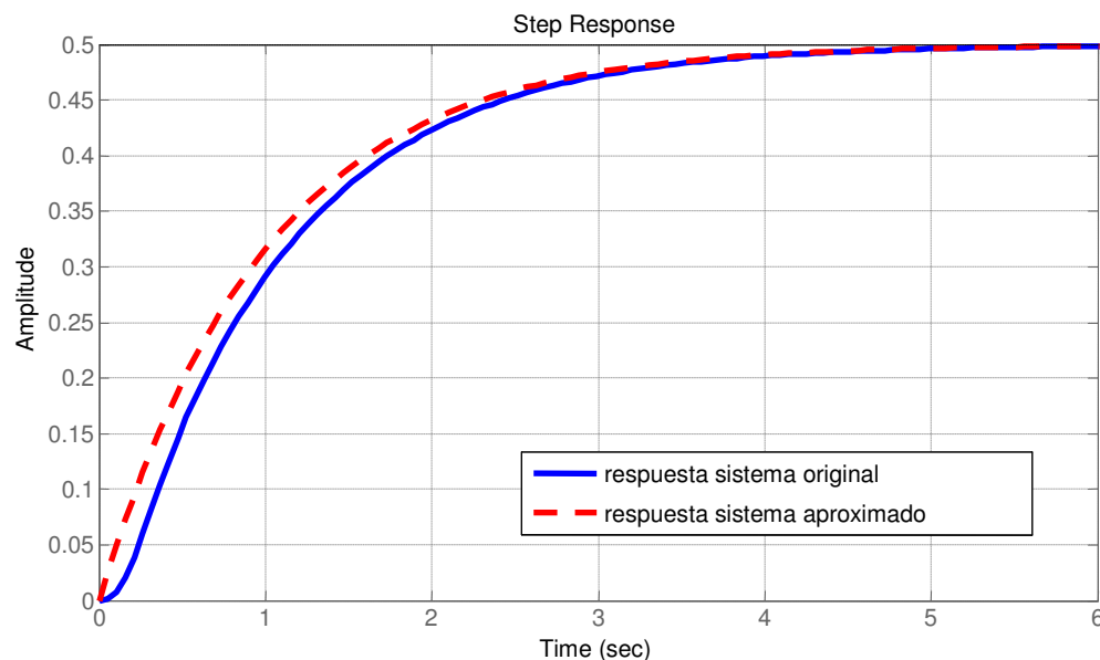
Figura 10.8.- Respuesta de un sistema dominante de primer orden.
