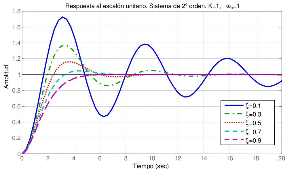
Figura 10.1.- Respuesta al escalón unitario de un sistema de 2º orden con diferentes factores de amortiguamiento (menores que 1).
