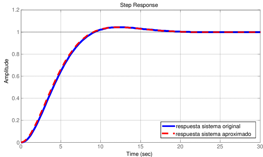
Figura 10.7.- Respuesta de un sistema dominante de segundo orden.
