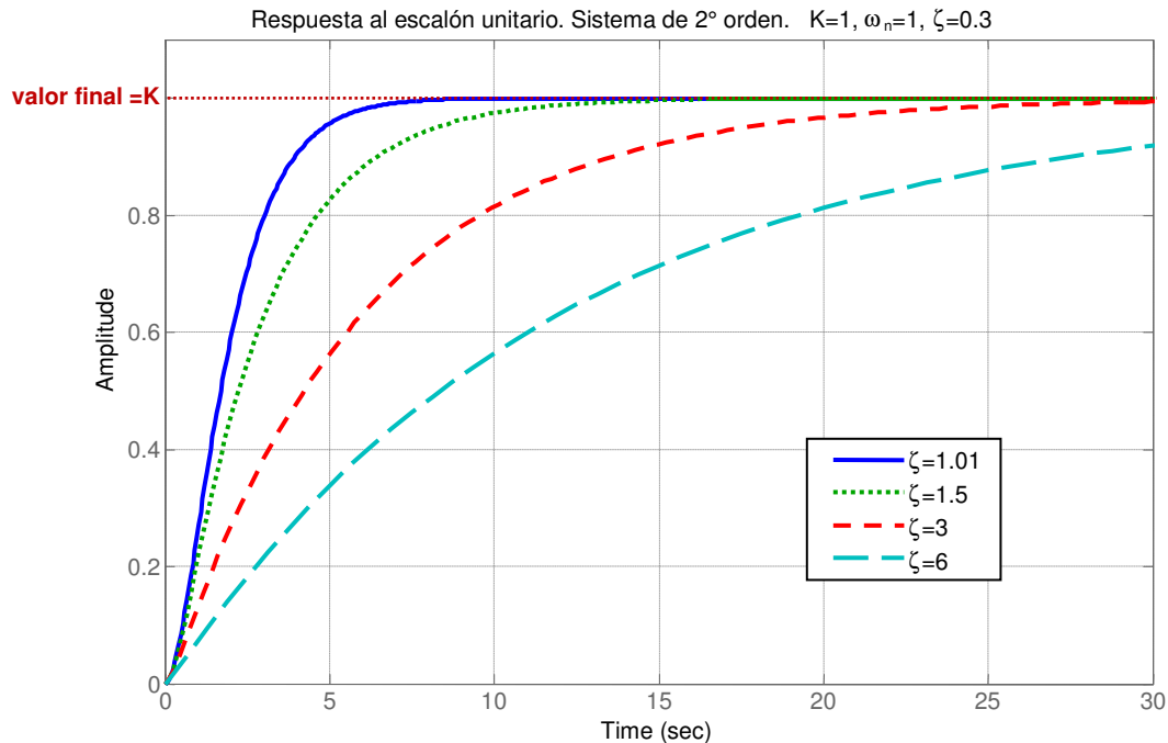
Figura 10.5.- Respuesta al escalón unitario en el caso sobreamortiguado de un sistema de 2° orden
