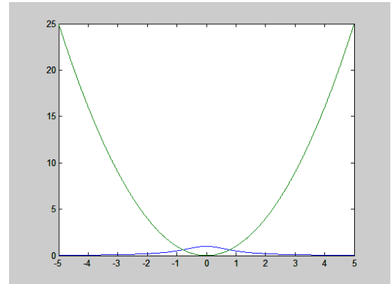
Figura 2.2 Parábola y curva de Agnesi
