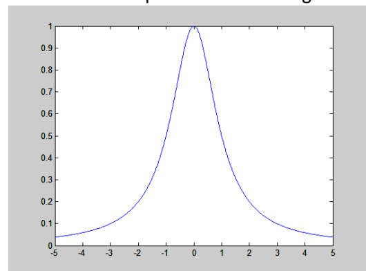
Figura 2.1 Curva de Agnesi
