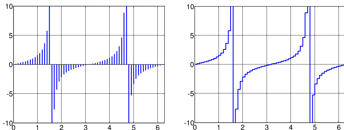
Figura 2.9 Gráficas de \tan(x) obtenidas mediante stem y stairs .
