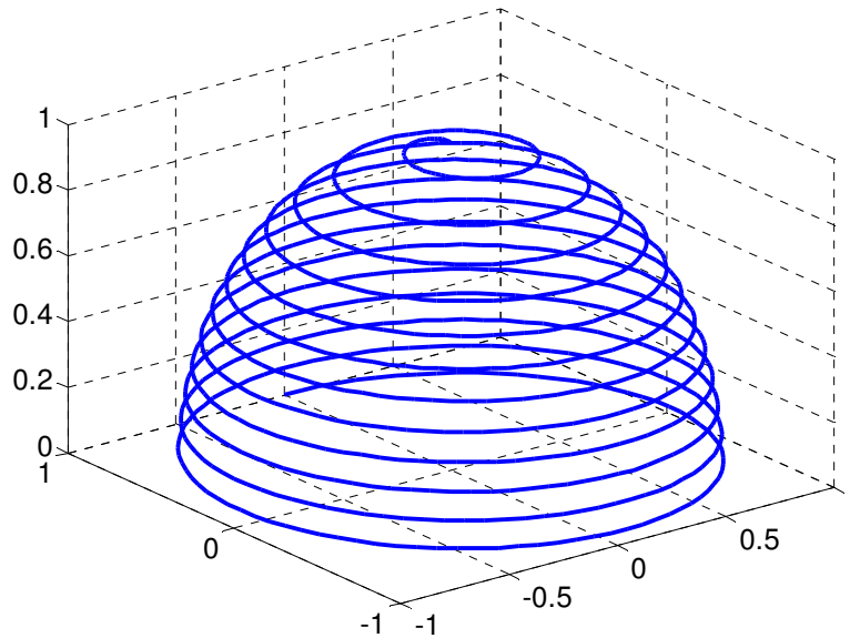
Figura 2.11. Ejemplo de línea tridimensional
