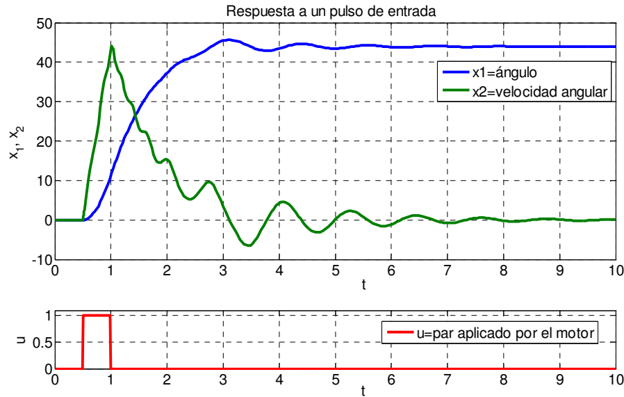
Figura 6.6.- Respuesta de la varilla a un pulso de par aplicado por el motor.
