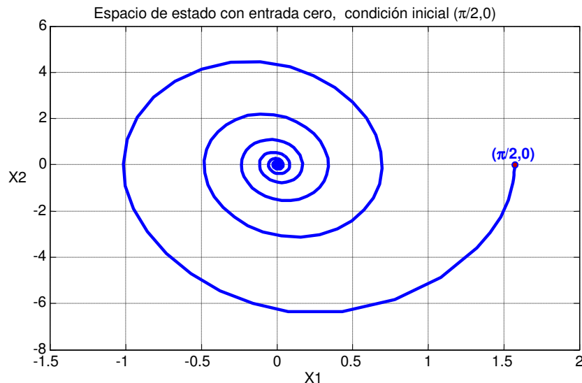
Figura 6.5.- Respuesta de la varilla sin actuador en el plano de estado.
