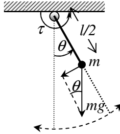
Figura 6.2.- Diagrama del cuerpo libre del centro de masa de la varilla.
