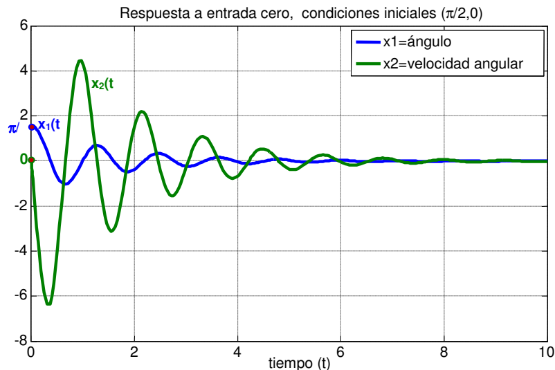
Figura 6.4.- Respuesta de la varilla con el actuador desconectado.
