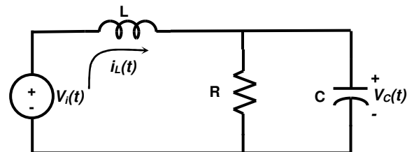
Figura 6.8.- Circuito para el problema 3 del reporte.
