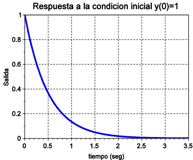
Figura 9.8.- Respuesta del sistema (9.10) a la condición inicial y(0) = 1
